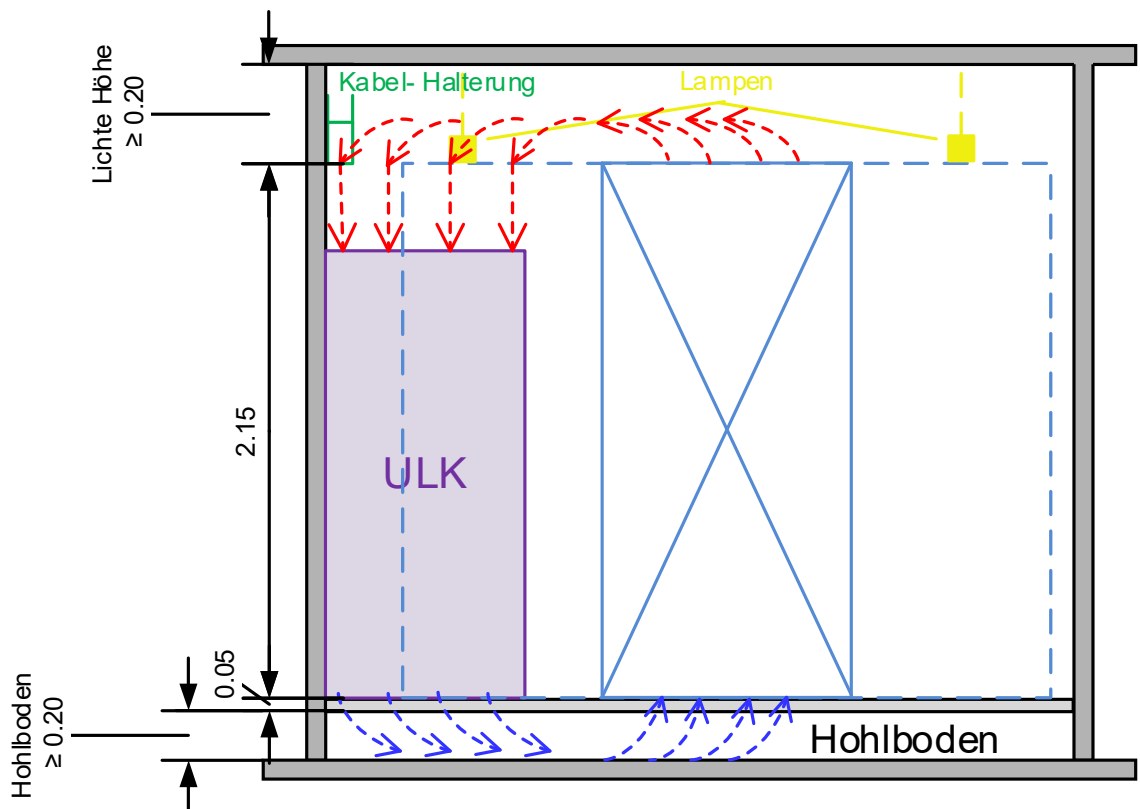
Abbildung 20 Raum Aufriss
