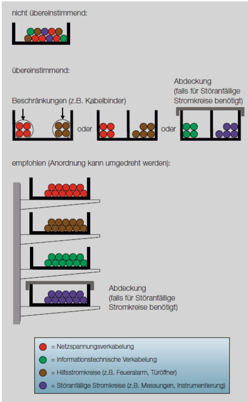
Abbildung 22 Trassebelegung
