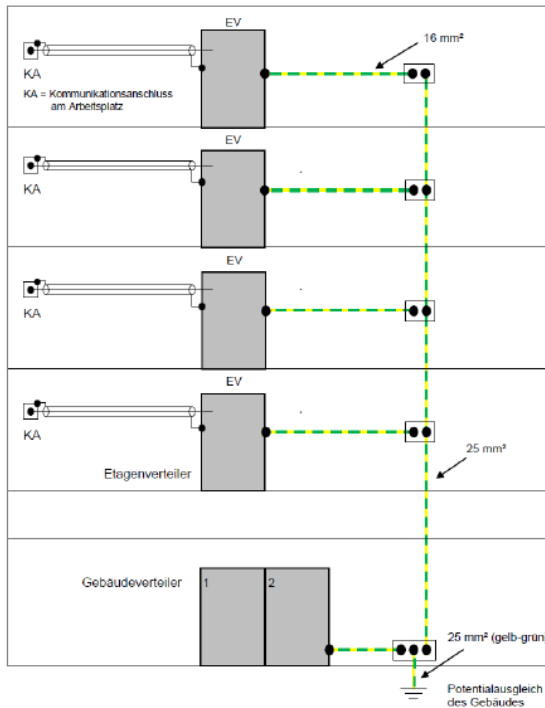
Abbildung 21 Erdungsprinzip
