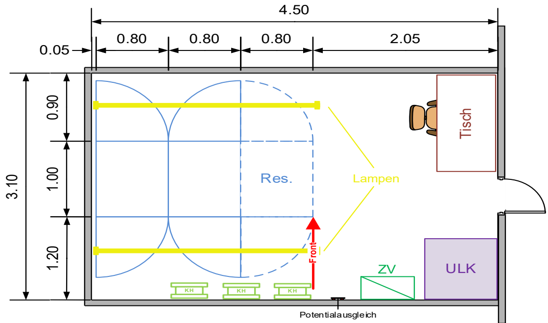
Abbildung 19 Raum Grundriss
