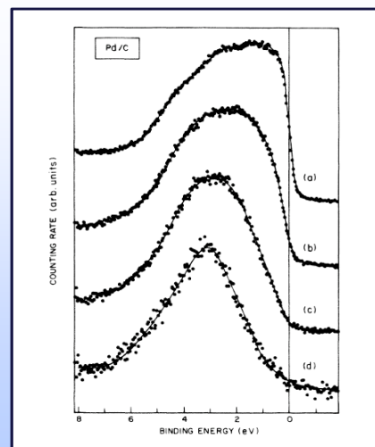
Bedeckung: a) bulk b) 4 \times 10^{15} c) 1 \times 10^{15} d) 3 \times 10^{14} atoms/cm 2
